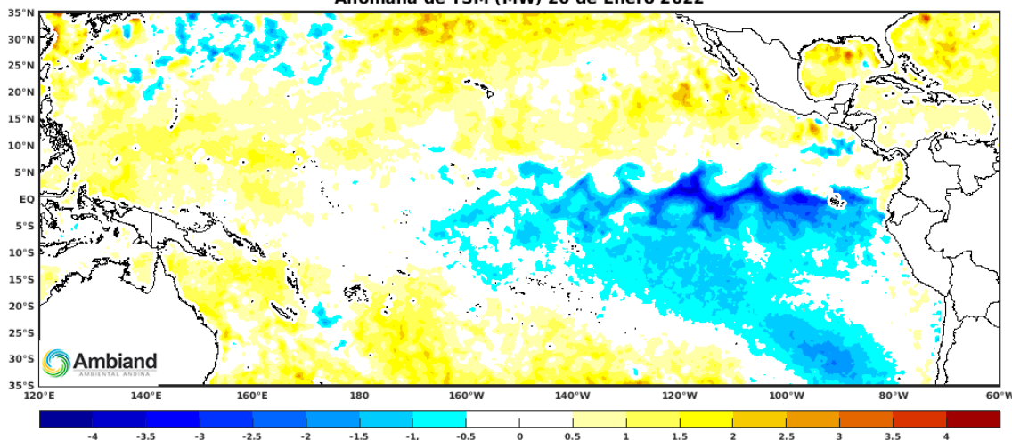
Anomalía de TSM (MW) 20 de Enero 2022
