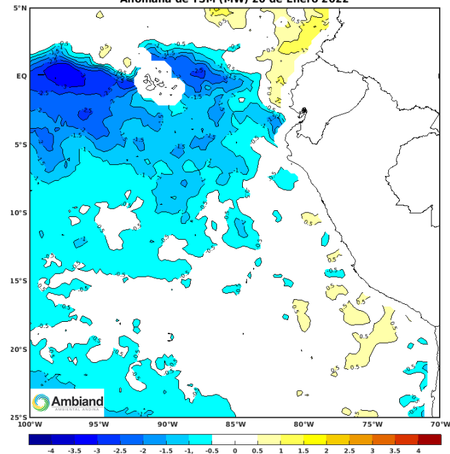
Anomalía de TSM (MW) 20 de Enero 2022
